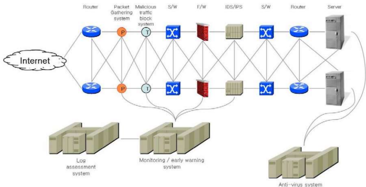
Surat 20. Toruň we ulgamlaryň strukturasynyň mysaly
