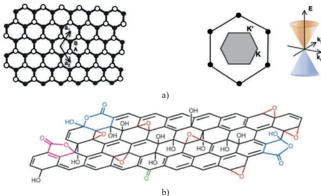
1-nji surat. Grafen oksidiniň yzygiderli geksagonal gurluşy (a) we onuň kislorod (-O) we gidroksil (-OH) toparlary bilen baglanyşygy (b)
