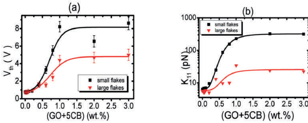
2-nji surat. Kiçi ( 0.56 \pm 0.32 mkm) we uly ( 2.8 \pm 1.6 mkm) ölçegli GO plitajyklarynyň 5CB suwuk kristal bilen dürli konsentrasiýaly garyndysynyň 25^\circ\text{C} temperaturadaky a) U_F Frederik geçiş naprýaženiýesi we b) maýyşgaklyk hemişeligi
