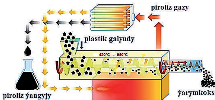
1-nji surat. Plastigi gaýtadan işläp bejermek üçin piroliz gurnawy
