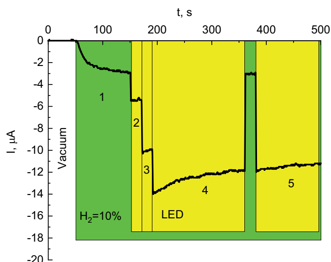
2-nji surat. 300 K-de 10 ob. % wodorod bilen gaz garyndysynda, tolkun uzynlygy 0,9 μm bolan, ýagtylyk diodynyň şöhlelenmesiniň dürli intensiwliginde ýşyklandyrylanda Pd/InP gurluşynda toguň generasiýasynyň kinetikasy. 1 – “wodorod togy”; 2, 3, 4 we 5 – “wodorod togunyň” we fototogunyň jemi; sary meýdan – ýagtylyk diody gurluşy ýşyklandyrýar. (ýagtylyk diody arkaly tok, mA: 1–0; 2–10; 3–30; 4 we 5–50); ýaşyl meýdan – gurluş wodorod gurşawynda ýerleşýär
