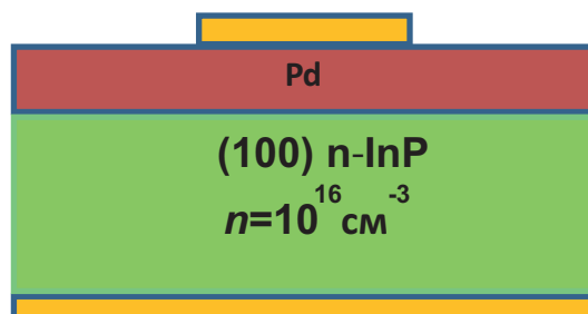
1-nji surat. Pd/InP gurluşynyň shemasy
