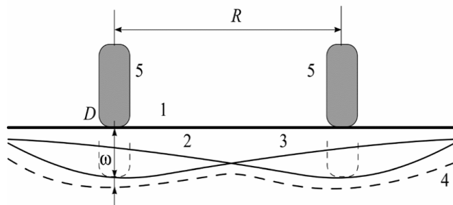
Рис.1 Схема деформирования дорожной конструкции при нагружении транспортным средством
