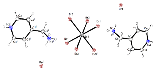
Рис.2. Структура \text{SnBr}_6 \cdot [\text{C}_6\text{N}_2\text{H}_{10}]^{+4} \cdot 2\text{Br}^{-2}
