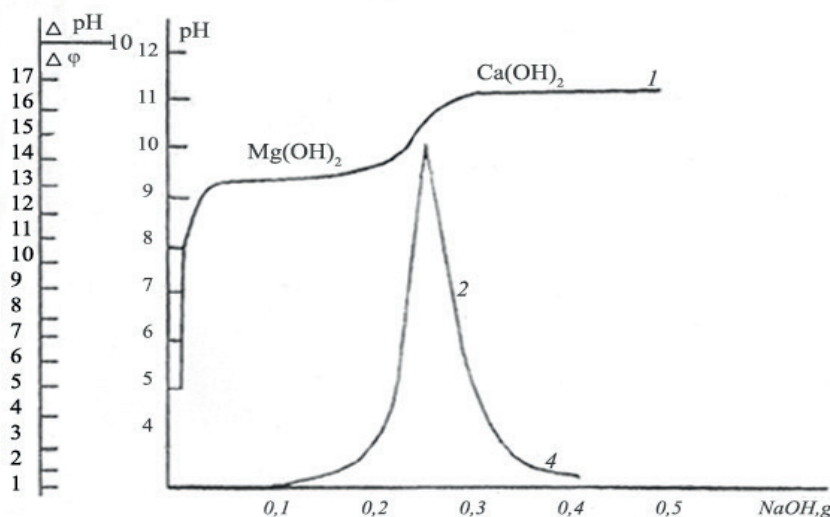
Рис. Потенциометрическая кривая осаждения ионов \text{Ca}^{2+} и \text{Mg}^{2+} в виде \text{Ca}(\text{OH})_2 и \text{Mg}(\text{OH})_2 при различном значении pH и добавлении NaOH
