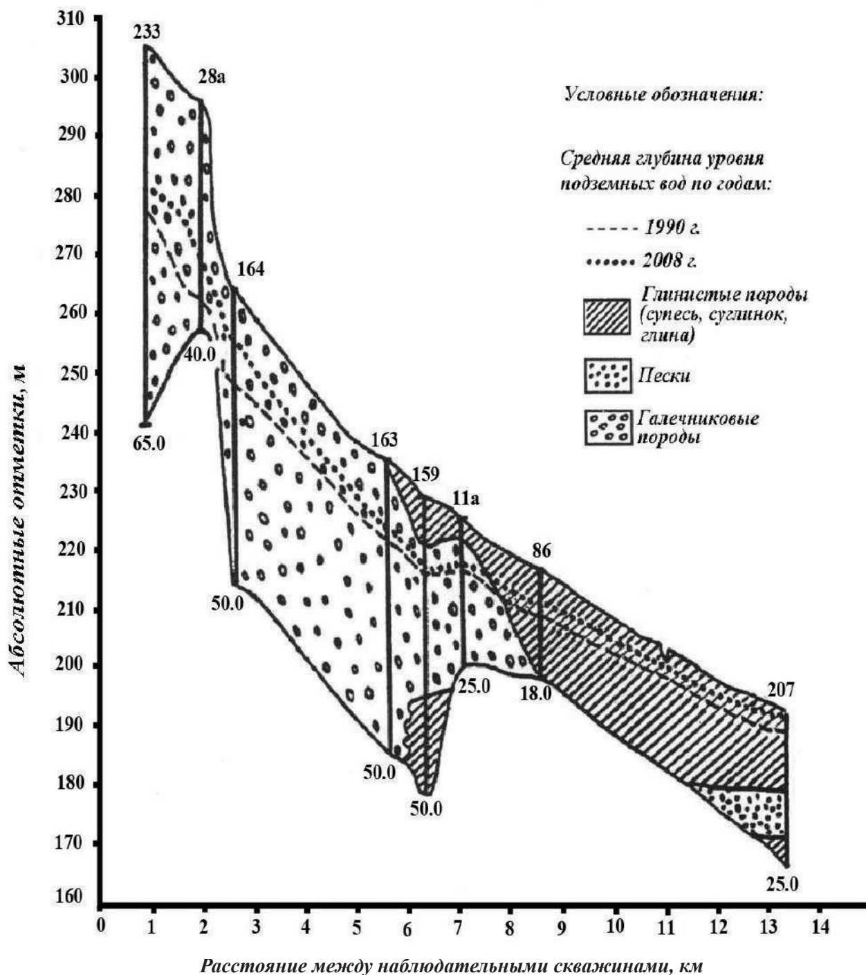
Рис. 2. Схематический гидрогеологический разрез территории г. Ашхабада с юга на север по наблюдательным скважинам
