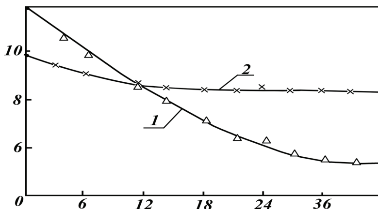
Рис. Изменение производительности трубчатых ультрафильтрационных (1) и обратноосмотических (2) полых волокон в процессе эксплуатации
