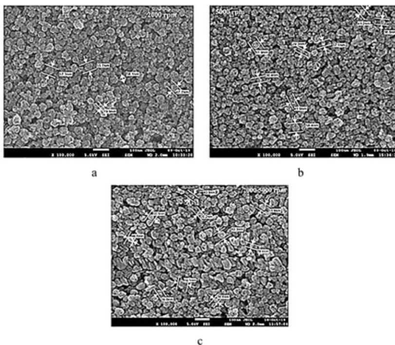
1-nji surat. Titan oksidiniň gatlagynyň üstüniň x 100.000 ulaldylan ýagdaýda: a) 2000 aýl/min; b) 5000 aýl/min; c) 2000-5000 aýl/min
