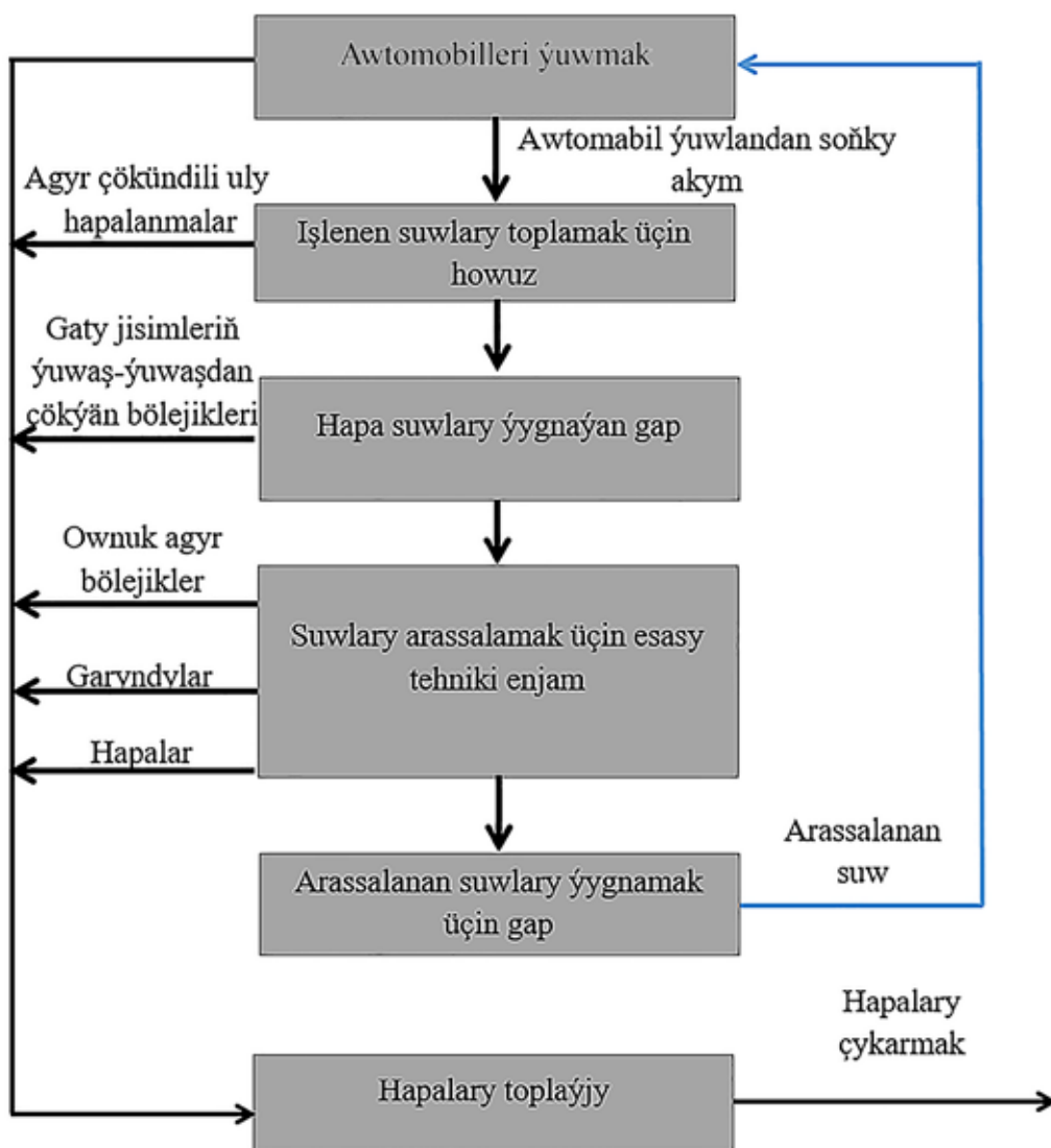
Awtomobiller ýuwalanda ulanylýan suwlaryň arassalanýş usullarynyň shemasy
