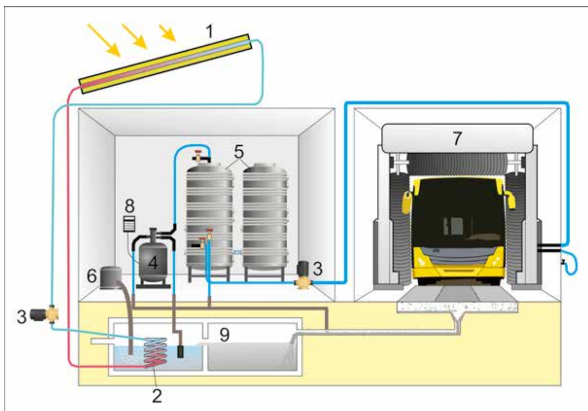
2-nji surat. Enjamyň gurluşynyň atlary: 1. Gün kollektory; 2. Gyzdyryjy spiral; 3. Nasos; 4. Filtirli nasos; 5. Suw bagy; 6. Arassalaýjy serisde; 7. Ýuwujy enjam; 8. Dolandyryjy gural; 9. Suwy arassalaýjy howuz (keselikdäki durlaýjy)
