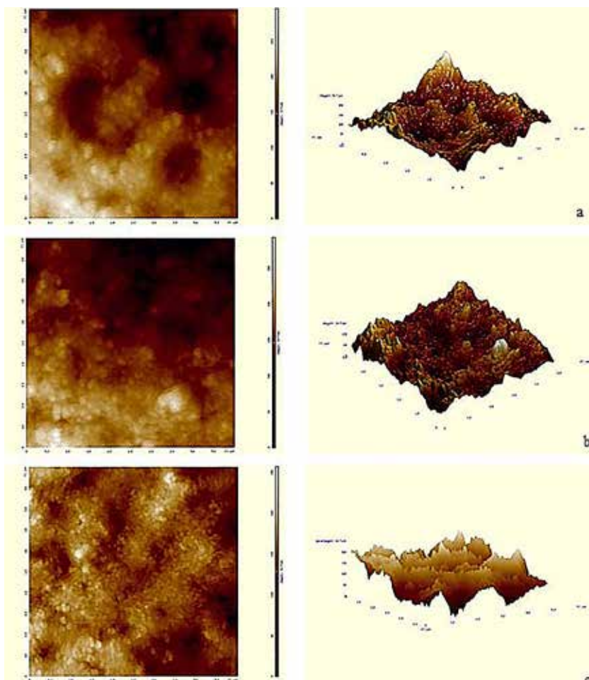
2-nji surat. Ölçegleriň 5 \times 5 \mu\text{m} bolan meýdanynyň üst topografiýasy we 3D suraty dürli aýlaw tizlikde: a) 2000 aýl/min; b) 5000 aýl/min; c) 2000-5000 aýl/min
