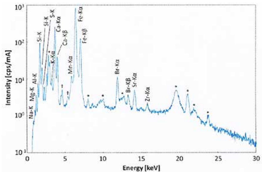
2-nji çyzgy. Mäne-Çäçäniň çäge nusgasynyň agyr fraksiýasynyň XRF derňewi
