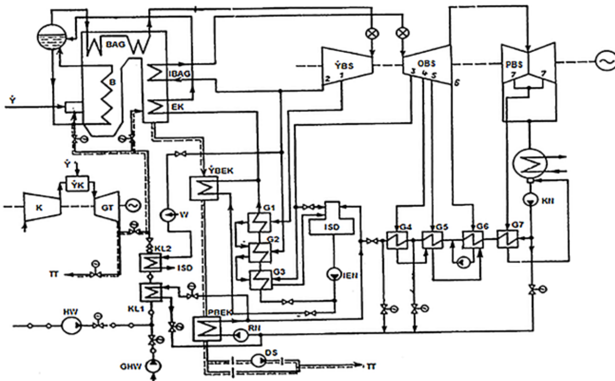
1-nji surat. Mary döwlet elektrik stansiýasynyň 8-nji energoblogynyň gaz turbina desgasy bilen utgaşykly dolanyşykda işletmegiň usuly.
